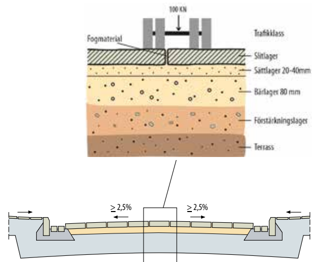
Fig 4.40 Uppbyggnad av väg bana belagd med hällar. Kantsten som motstöd.
