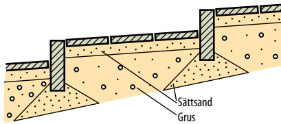
Fig 7.24 Åsnestig med sättsteg av kantsten och plansteg av hällar.
