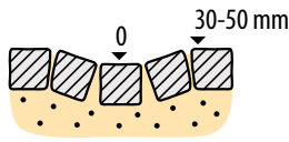
Fig 5.15 Rännsten, satt med 3 rader storgatsten
